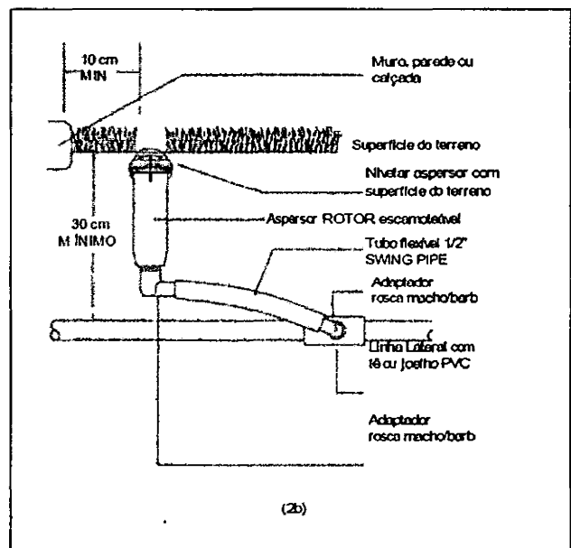
FIGURA 2: Detalhes de montagem dos aspersores escamoteáveis SPRAY (2a) e ROTOR (2b), com sistema flexível.
