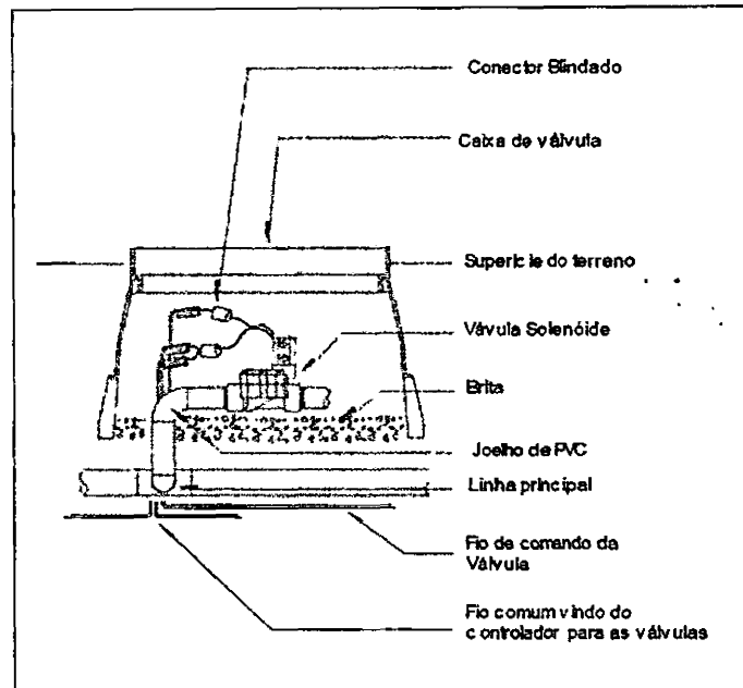
FIGURA 4: Detalhe de instalação da válvula solenóide
