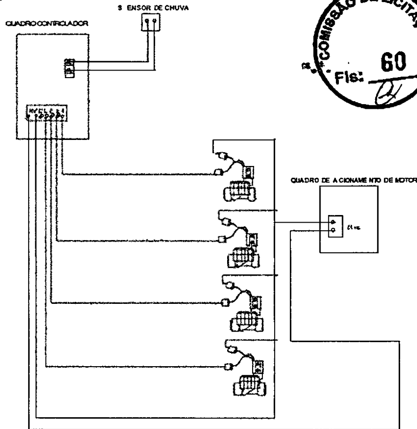
FIGURA 5: Detalhe de instalação do quadro controlador
