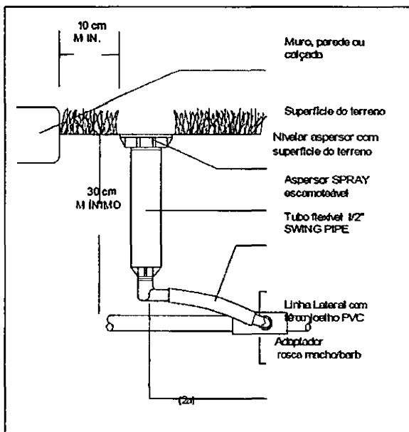
FIGURA 2: Detalhes de montagem dos aspersores escamoteáveis SPRAY (2a) e ROTOR (2b), com sistema flexível.
